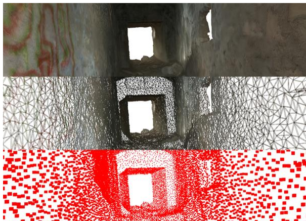
Figura 6: De arriba abajo: textura, malla de alambre y nube de puntos del interior del túnel del búnker.
